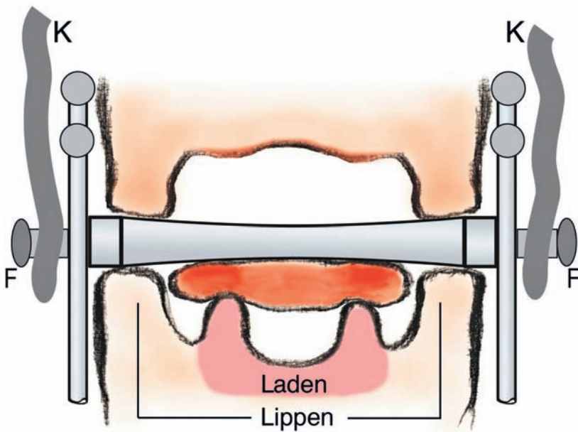
Abb. 2: Technisch vorteilhafte Aufhängung der Kandare. Die Kopfriemen K werden in die pilzförmigen Fortsätze F der Stange eingeknüpft. So bleibt die Höhenposition der Stange konstant
